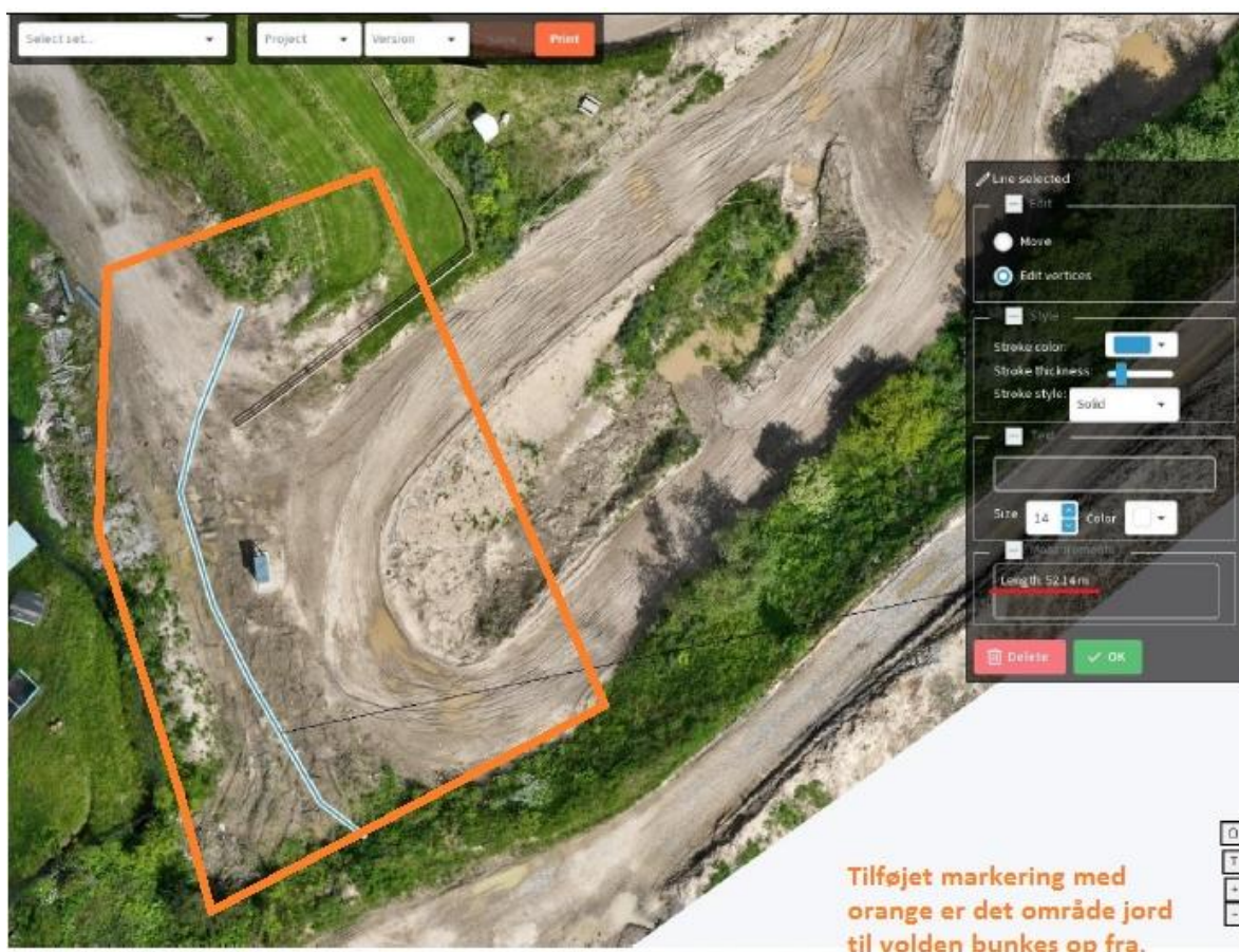
Skitse med mål på længde af ny vold. Opmålt via byggepladsen.dk
