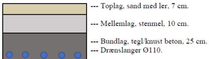
2 - Snit der viser opbygningen af ridebanen.
