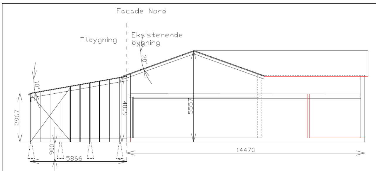
2 - Facadetegning af den nordlige facade.
