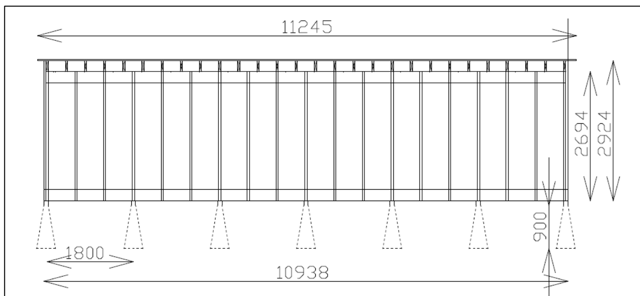
4 - Facadetegning af den østlige facade.
