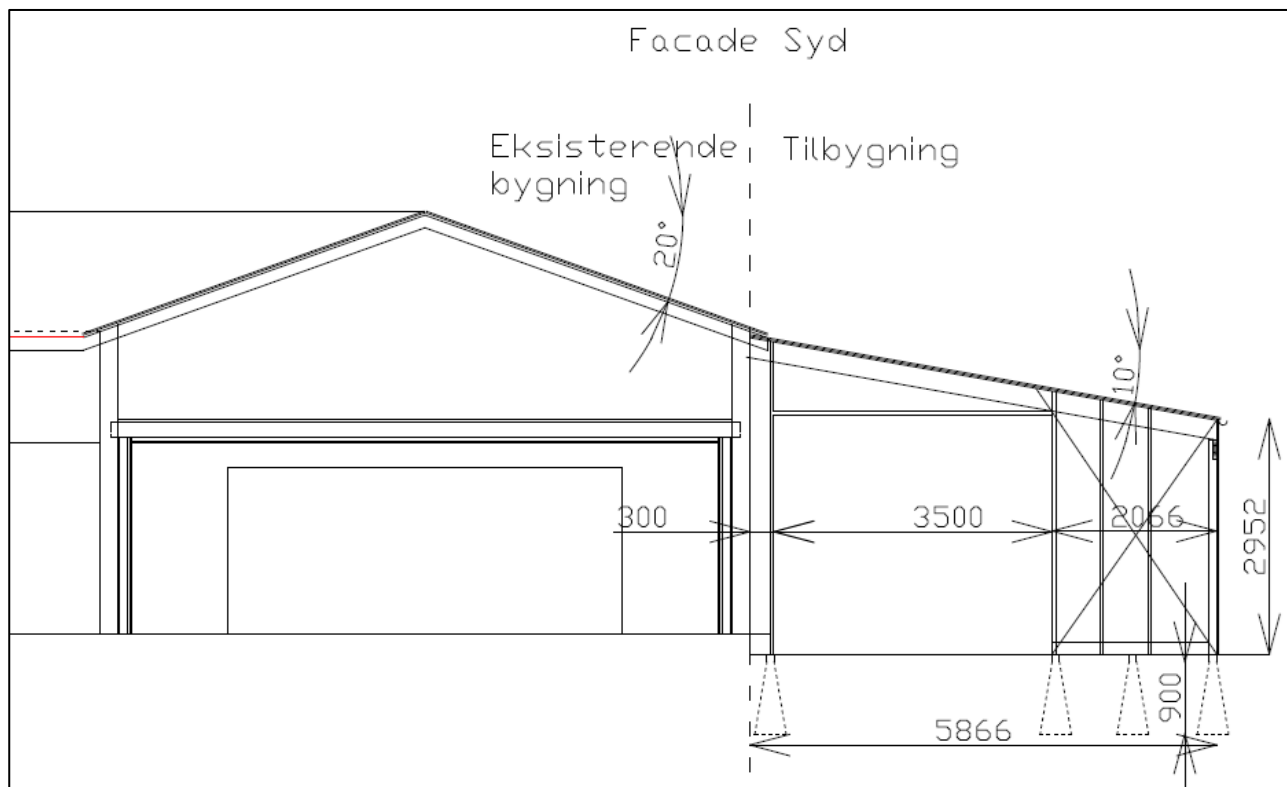
3 - Facadetegning af den sydlige facade.
