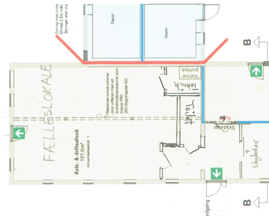
2 - Plantegning af det ansøgte mødelokale.
