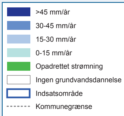
Figur 8b. Beregnet grundvandsdannelse til kildepladser i S1 og P1
