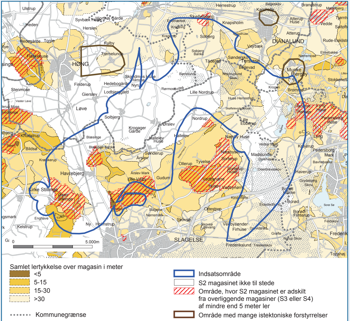
Figur 4. Geologisk beskyttelse af øvre Tude Å Magasin (S2).
