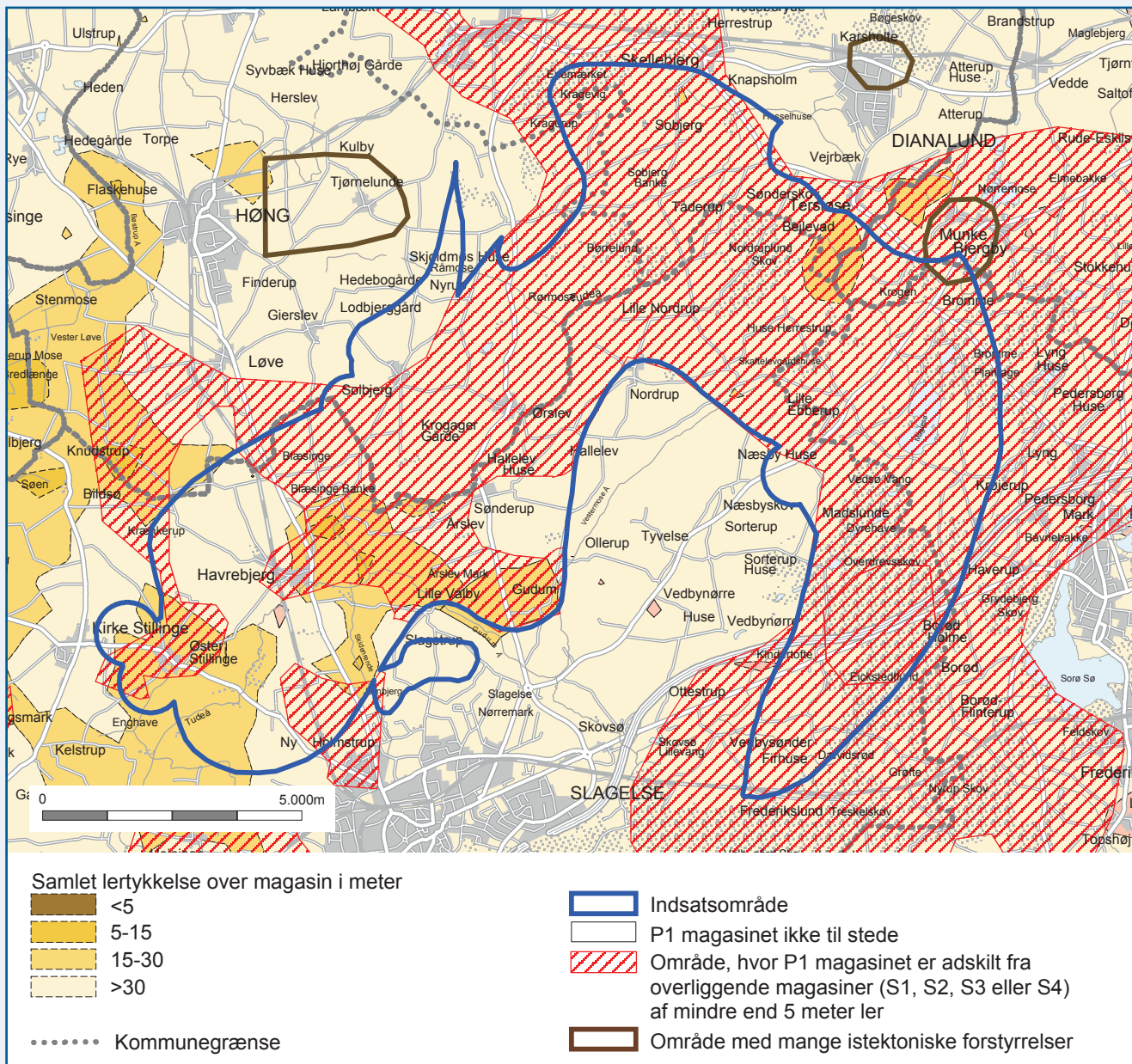
Figur 6. Geologisk beskyttelse af nedre Tude Å magasin (det prækvartære magasin P1).
